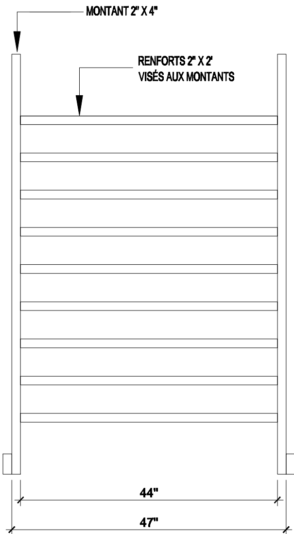
ÉLÉVATION A ÉCHELLE 3/4" = 1'-0"
