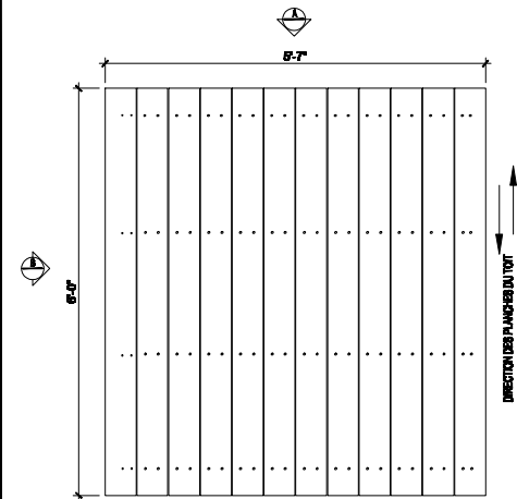
PLAN DU TOIT FINI ÉCHELLE 1/2" = 1'-0"
