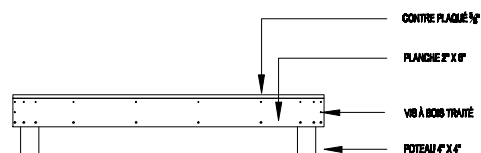
ÉLÉVATION A ÉCHELLE 1/2" = 1'-0"
