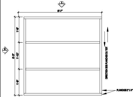
PLAN DU TOIT ÉCHELLE 1/2" = 1'-0"
