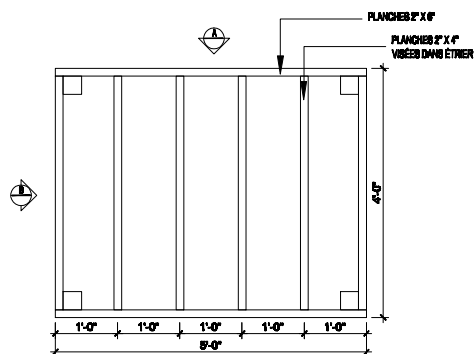
PLAN DE LA BASE ÉCHELLE 1/2" = 1'-0"
