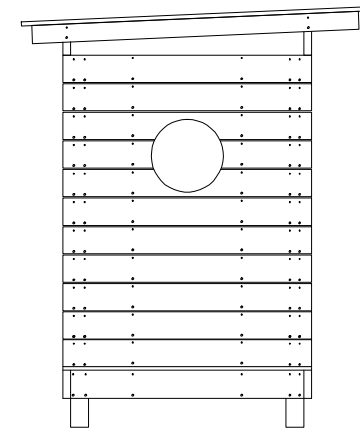
ÉLÉVATION CABANE ENFANT FINI ÉCHELLE 1/2" = 1'-0"
