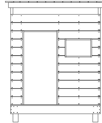
ÉLÉVATION CABANE ENFANT FINI ÉCHELLE 1/2" = 1'-0"
