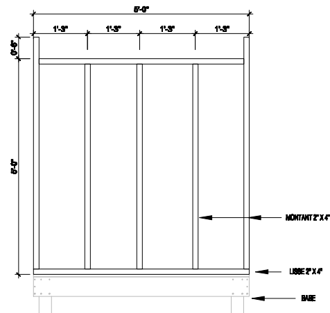
ÉLÉVATION MUR DE DERRIÈRE ÉCHELLE 1/2" = 1'-0"
