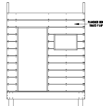
ÉLÉVATION MUR AVANT FINI ÉCHELLE 1/2" = 1'-0"
