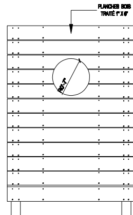
ÉLÉVATION 2 MURS LATÉRAUX FINIS ÉCHELLE 1/2" = 1'-0"
