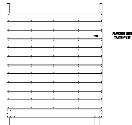
ÉLÉVATION MUR DE DERRIÈRE FINI ÉCHELLE 1/2" = 1'-0"
