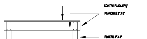
ÉLÉVATION B ÉCHELLE 1/2" = 1'-0"
