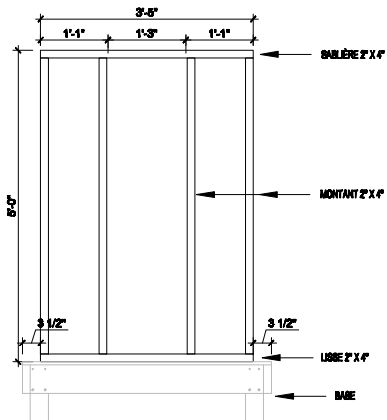
ÉLÉVATION 2 MURS LATÉRAUX ÉCHELLE 1/2" = 1'-0"
