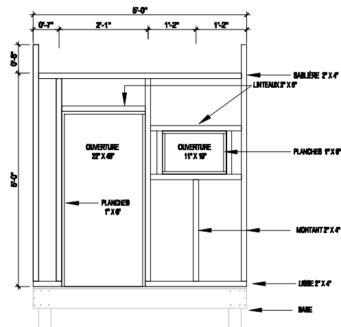
ÉLÉVATION DU MUR AVANT ÉCHELLE 1/2" = 1'-0"
