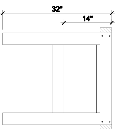
ÉLÉVATION B TABLE ÉCHELLE 3/4" = 1'-0"
