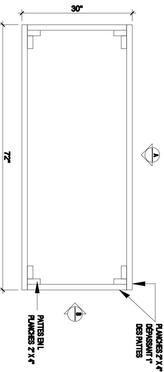
PLAN DE BASE DU BÂTI ÉCHELLE 3/4" = 1'-0"
