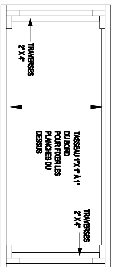
PLAN DE BASE ÉCHELLE 3/4" = 1'-0"
