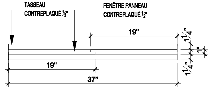
DÉTAIL FENÊTRE PLAN ÉCHELLE 1" = 1'-0"
