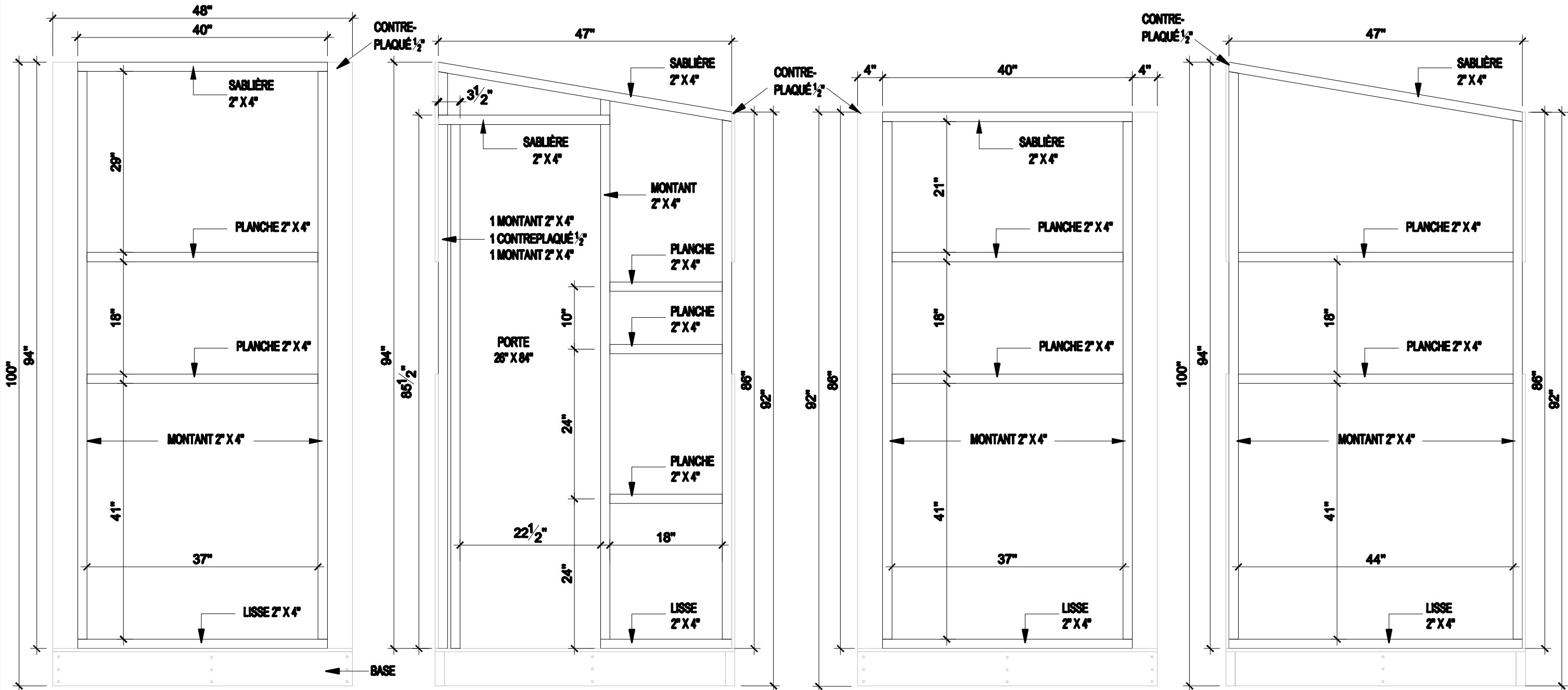
ÉLÉVATION A MUR DU FOND
