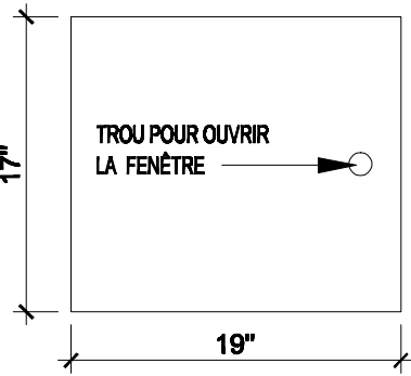
FENÊTRE DEVANT ET FOND ÉCHELLE 1" = 1'-0"
