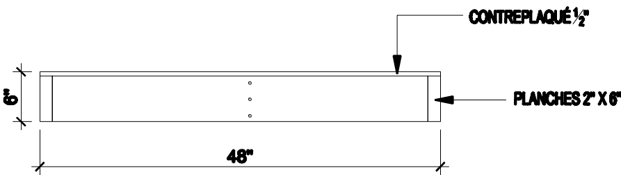
ÉLÉVATION B DE LA BASE ÉCHELLE 3/4" = 1'-0"
