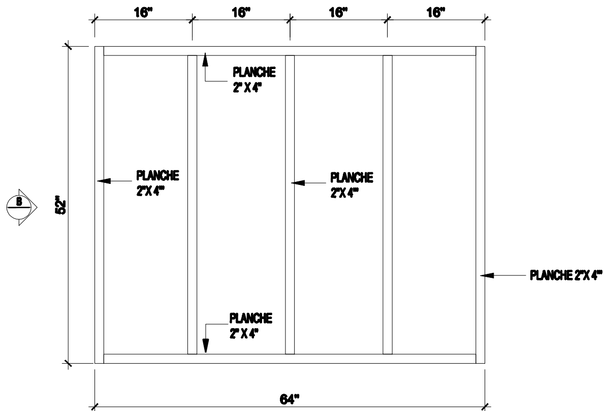
PLAN DU TOIT ÉCHELLE 3/4" = 1'-0"
