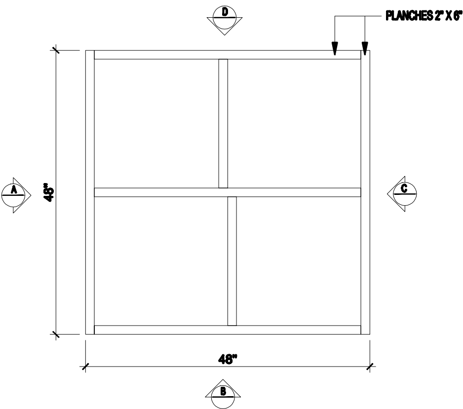
PLAN DE LA BASE ÉCHELLE 3/4" = 1'-0"
