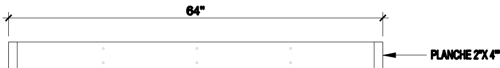
ÉLÉVATION A ÉCHELLE 3/4" = 1'-0"
