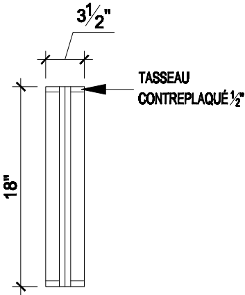
DÉTAIL FENÊTRE ÉLEVATION ÉCHELLE 1" = 1'-0"
