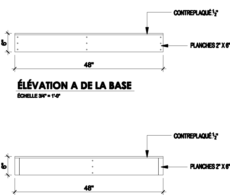
ÉLÉVATION B DE LA BASE ÉCHELLE 3/4" = 1'-0"
