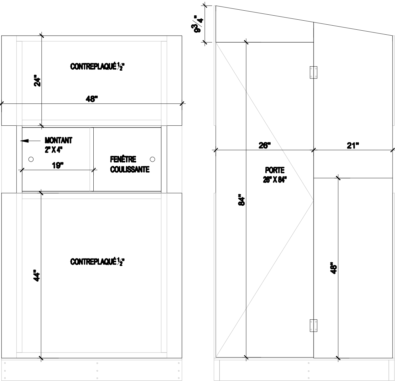
ÉLEVATION MUR DEVANT ÉCHELLE 3/4" = 1'-0"
