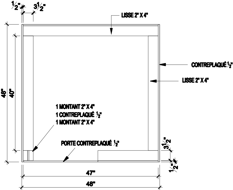
PLAN DES MURS ÉCHELLE 3/4" = 1'-0"
