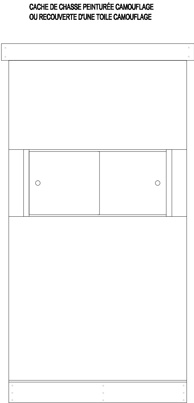
CACHE DE CHASSE FINIE ÉCHELLE 3/4" = 1'-0"
